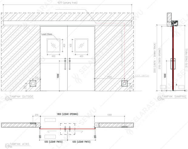
HERMETIC DOUBLE
